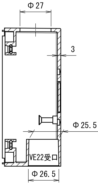
断面 A-A
